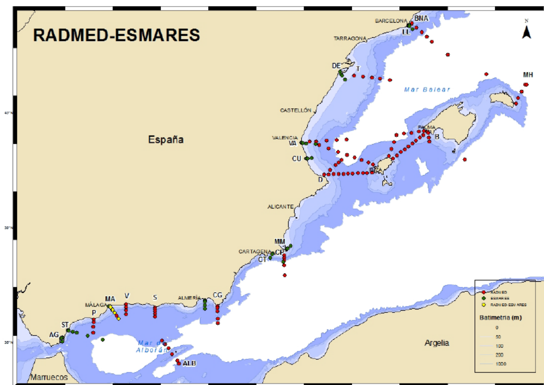
Mapa donde figuran todas las estaciones: (P: Cabo Pino; M: Málaga; V: Vélez-Málaga; S: Cabo Sacratif; CG: Cabo de Gata; CP: Cabo Palos; D: Denia; GV: Golfo Valencia; T: Tarragona; BNA: Barcelona; B: Baleares; MH: Mahón; ALB: Alborán). ESMARES (AG: Algeciras; ST: Sotogrande; MA: Málaga; AL: Almería; CT: Cartagena; MM: Mar Menor; CU: Cullera; VA: Valencia; DE: Delta del Ebro; LL: Llobregat).
